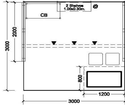
LAY-OUT PLAN
